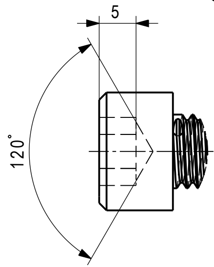
Détail B Echelle : 2:1
